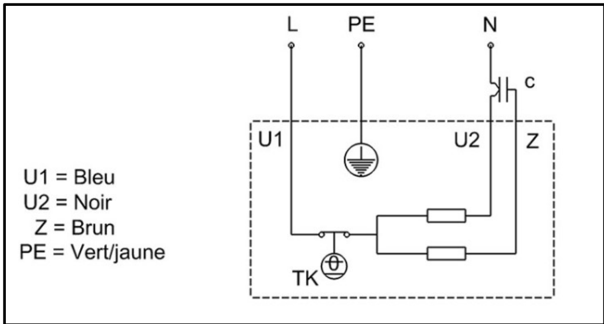
Kopplingschema TAK250-1415AC
