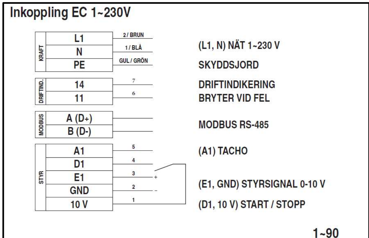
Kopplingschema TAK 280-2040, 355-1550
